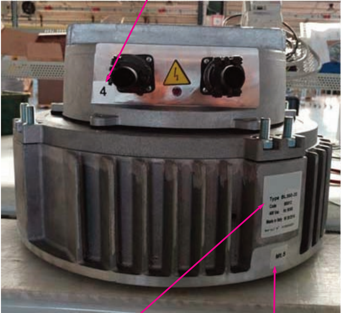
Etikette Modell, Motoinverter und Serial Number
